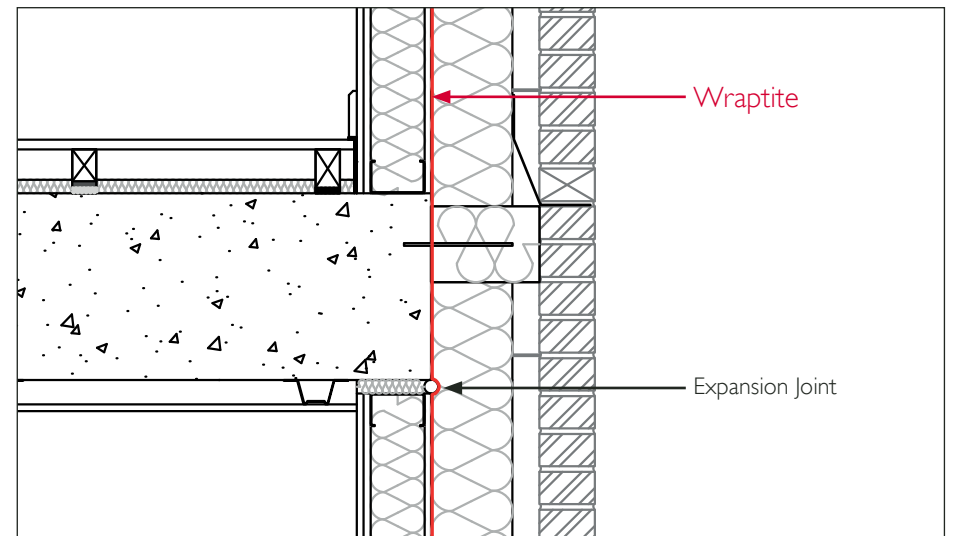
SLAB EDGE - BRICK FAÇADE
